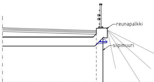
Kuva 3. Kaapelireitin sijoitus laattakehäsilltaan, jossa on ylittävän väylän suuntaiset siipimuurit. Suoja-putket jatkuvat penkereeseen.
